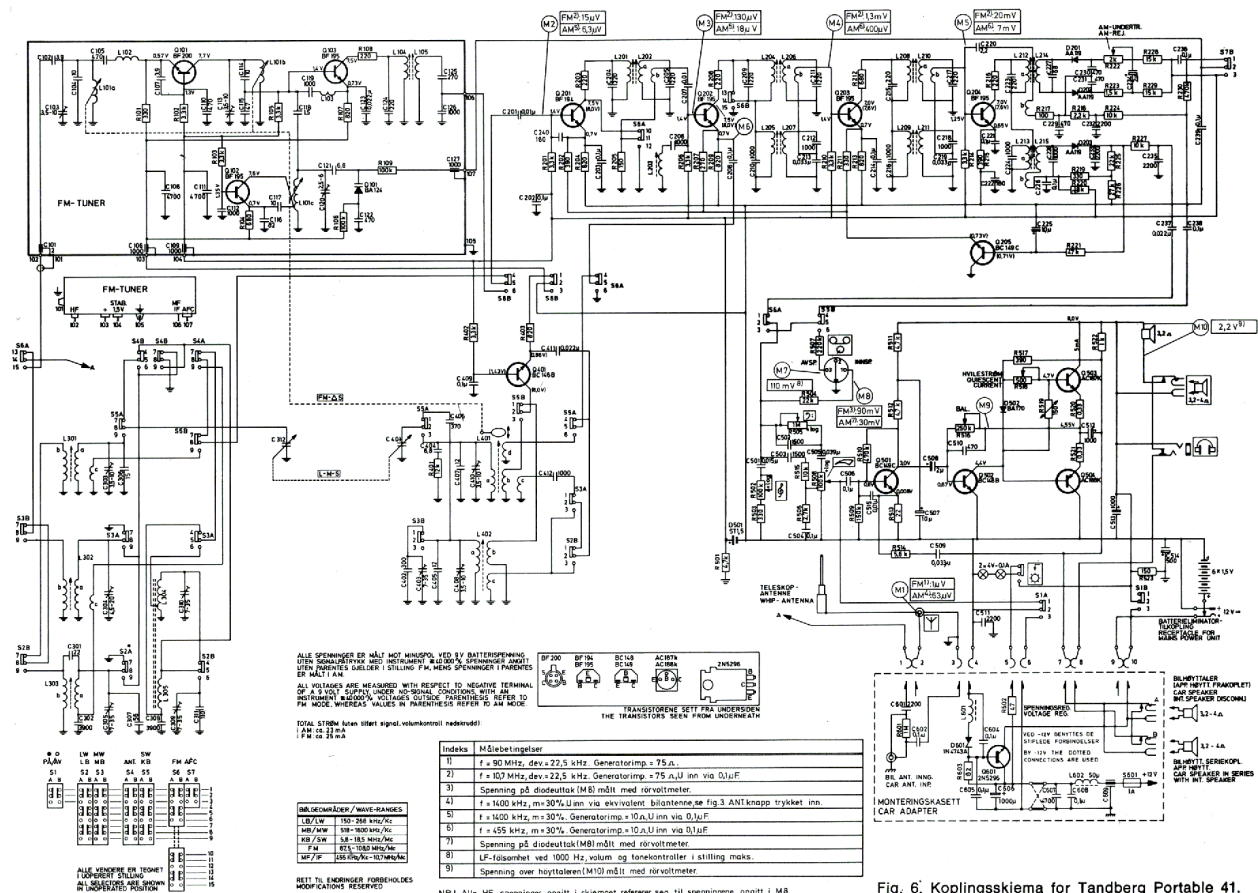
Fig. 6. Koplingskjema for Tandberg Portable 41.
